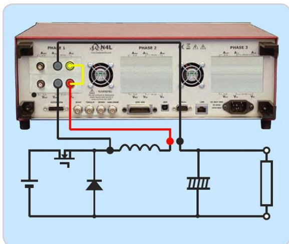
Схема измерения
